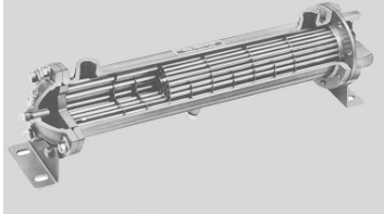
水冷冷却器
