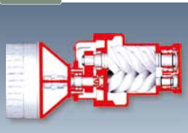
联轴器
